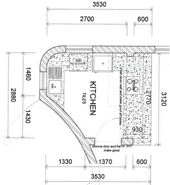
LAYOUT : UNIT 18 & 19 SCALE 1:50
