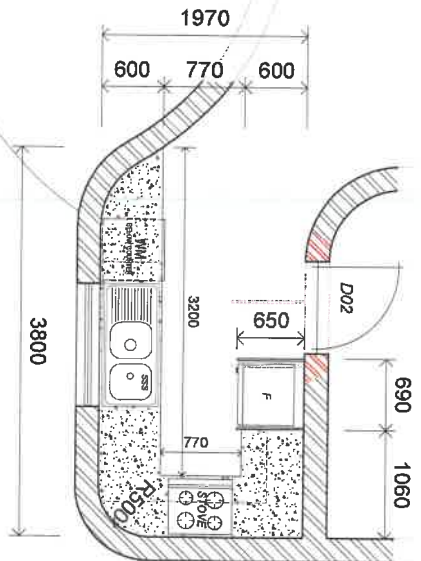
LAYOUT : UNITS 01 - 14 SCALE 1:50
